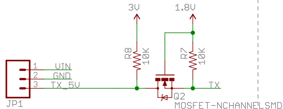
I/O Section
